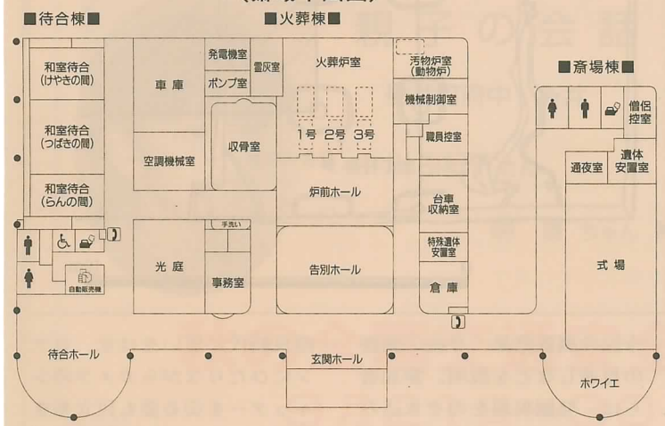
〈斎場平面図〉
