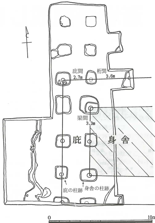
御旅神社西側遺構実測図
